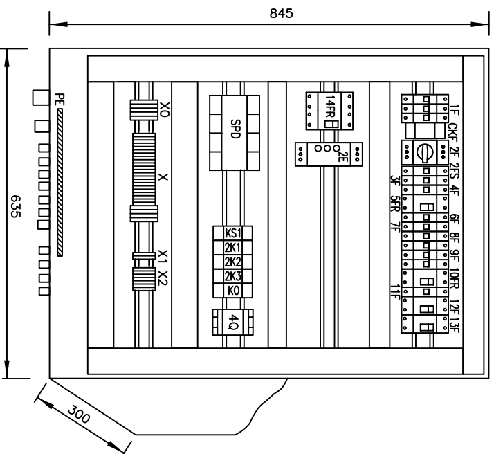
WIDOK WNIĘTRZA
