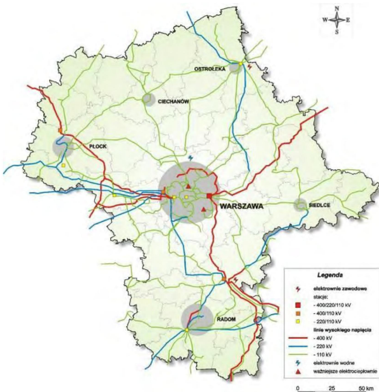
Rysunek 14. Przebieg linii elektroenergetycznych w woj. mazowieckim (na podstawie Planu Zagospodarowania Przestrzennego Województwa Mazowieckiego).
